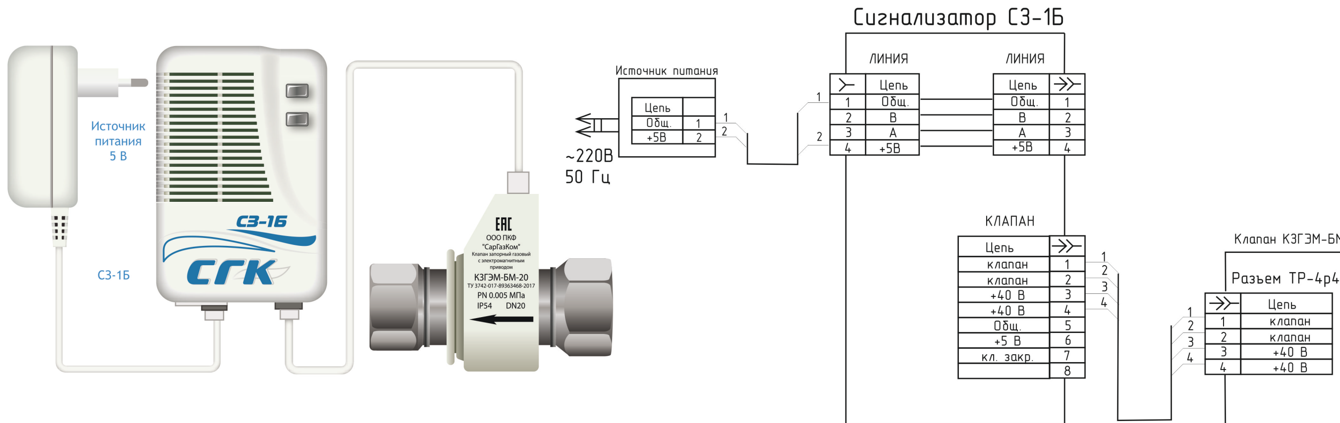
Система автономного контроля загазованности СГК-1-Б-СН с клапаном КЗГЭМ-БМ
